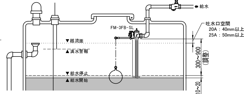
■ 設置例図
