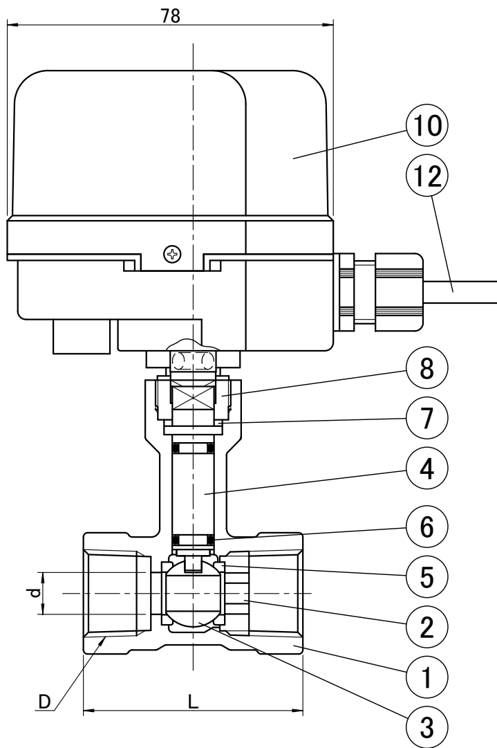
■ 寸法表
