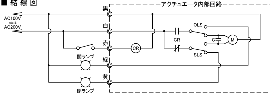
■ 結線図
