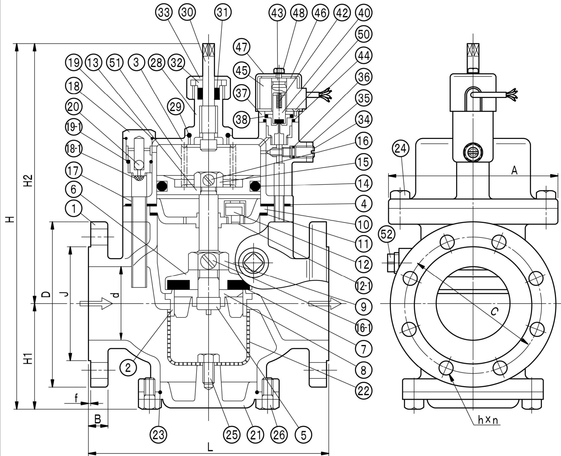
■ 寸法表
